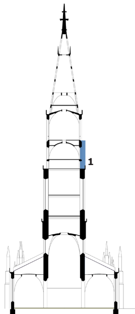
Querschnitt
